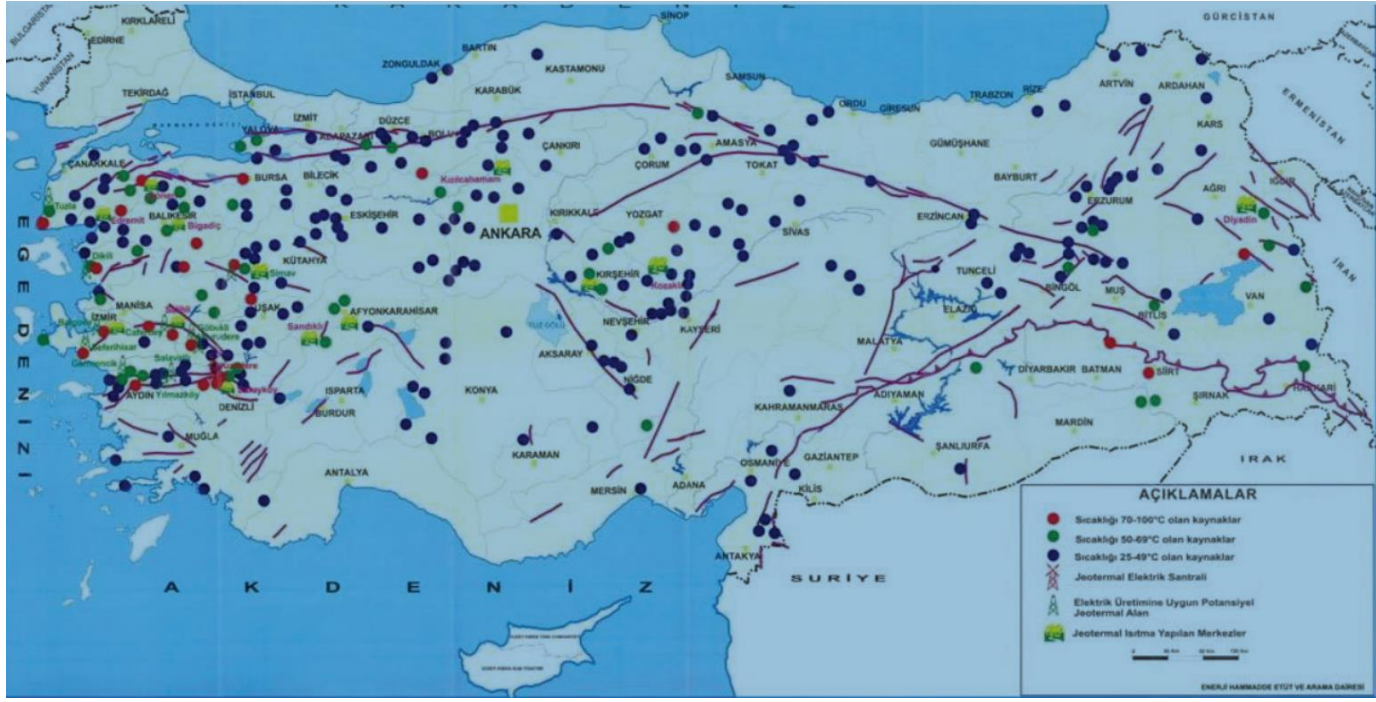
Figure 1. Türkiye'nin Jeotermal Kaynak Haritası
